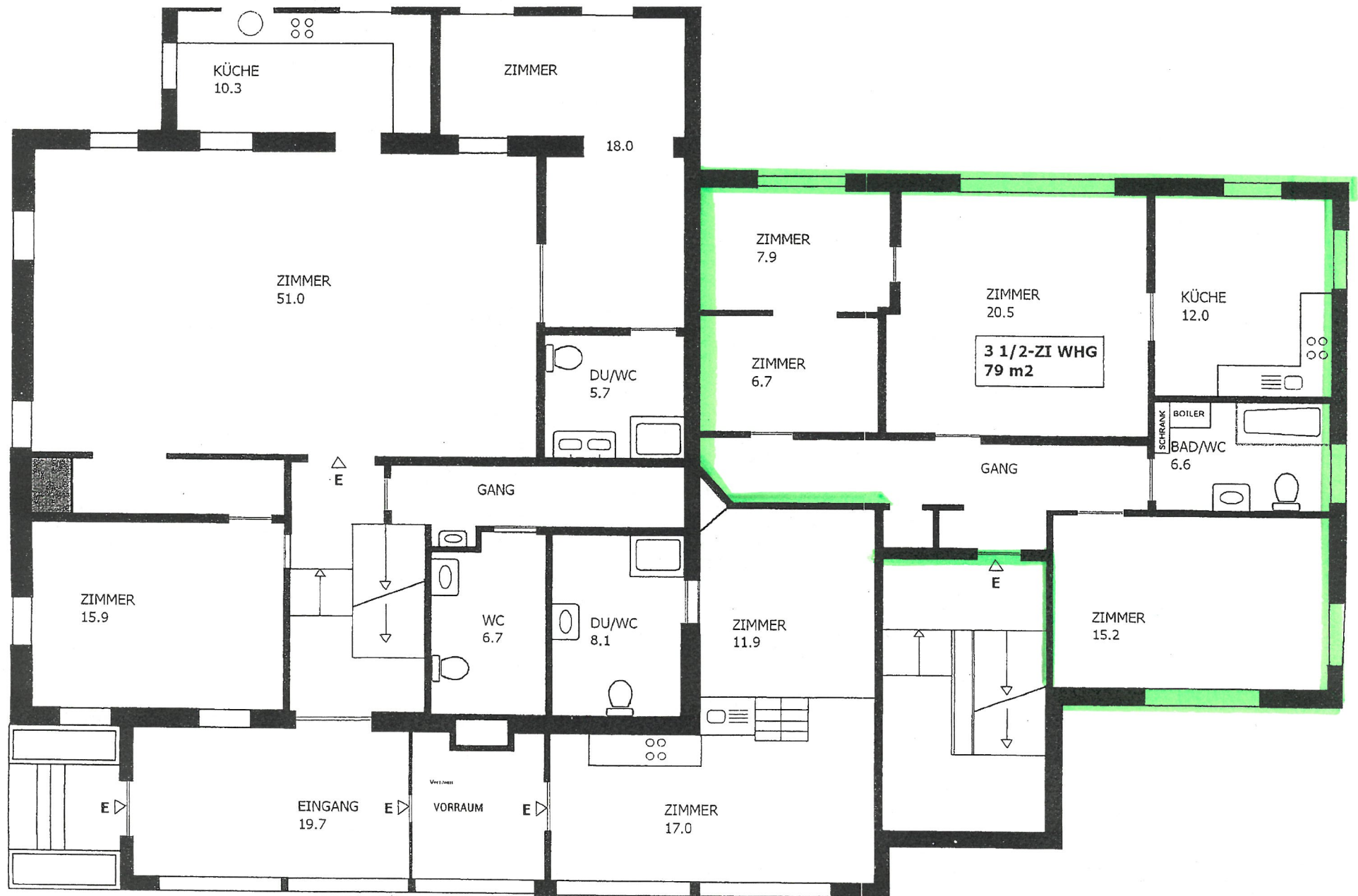
1. OBERGESCHOSS
