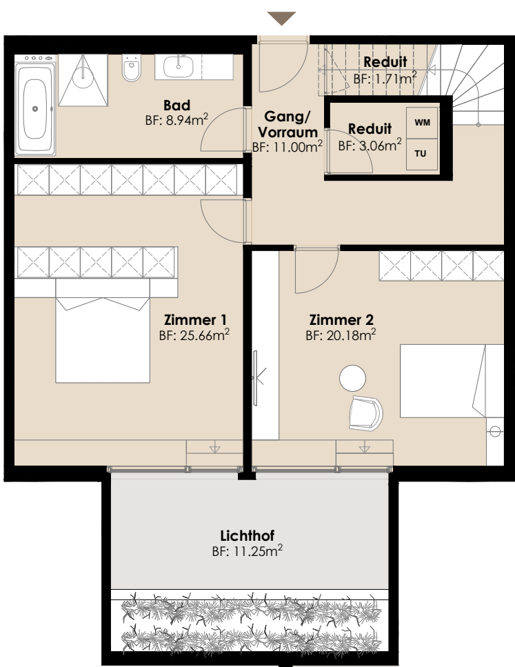
_Sockelgeschoss
