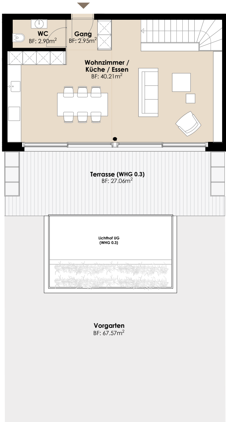
_Erdgeschoss
