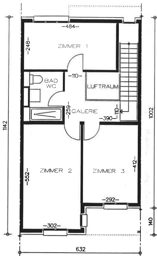
1. OBERGESCHOSS
