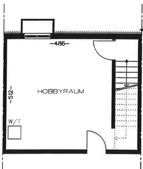
UNTERGESCHOSS
