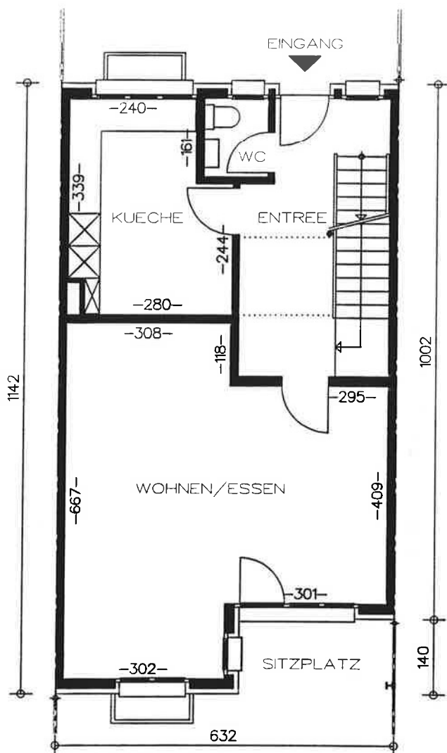
ERDGESCHOSS
