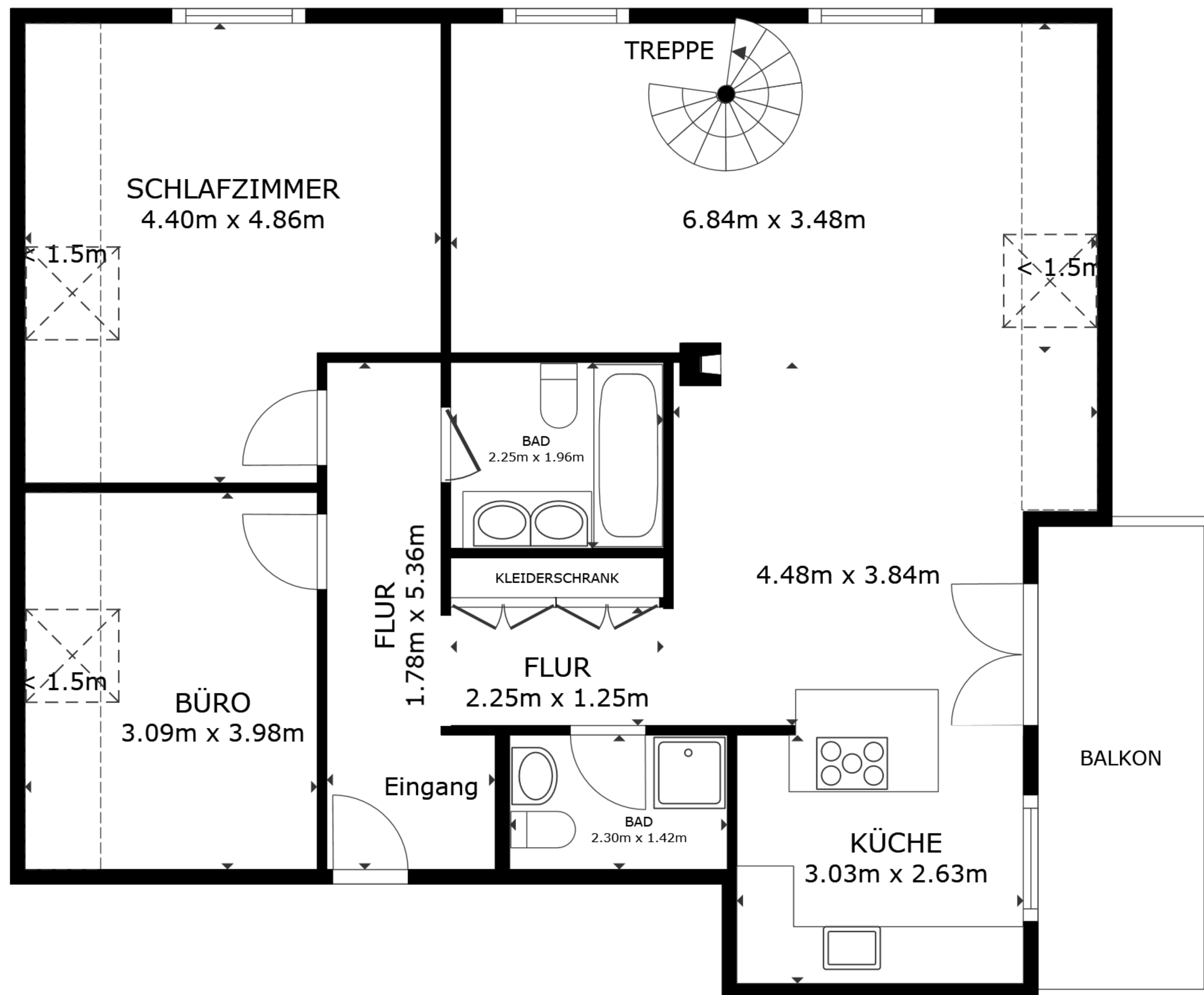
STOCKWERK 1
