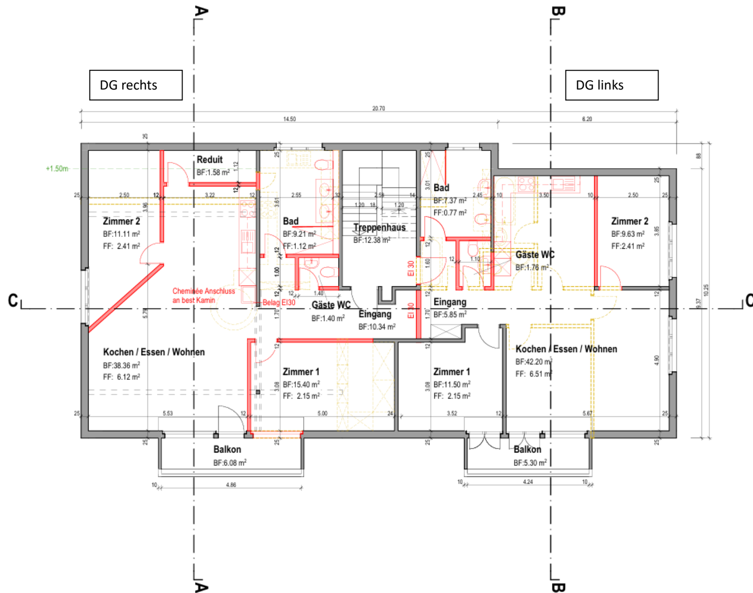
Grundriss Dachgeschoss
