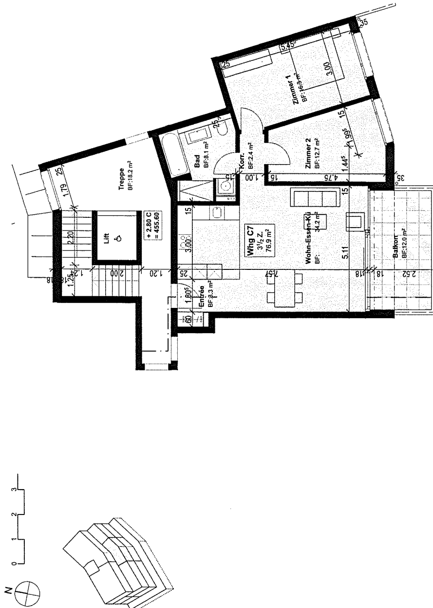
3 MFH mit Einstellhalle, Santelstrasse Egerkingen
