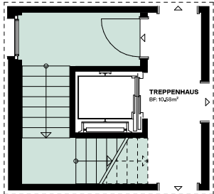
Ausschnitt OG 2
