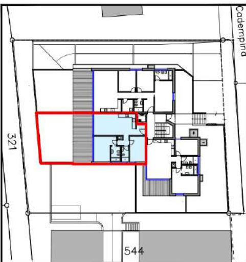
Pianterreno 1:100
