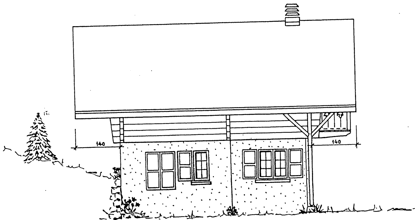
FAÇADE OUEST
