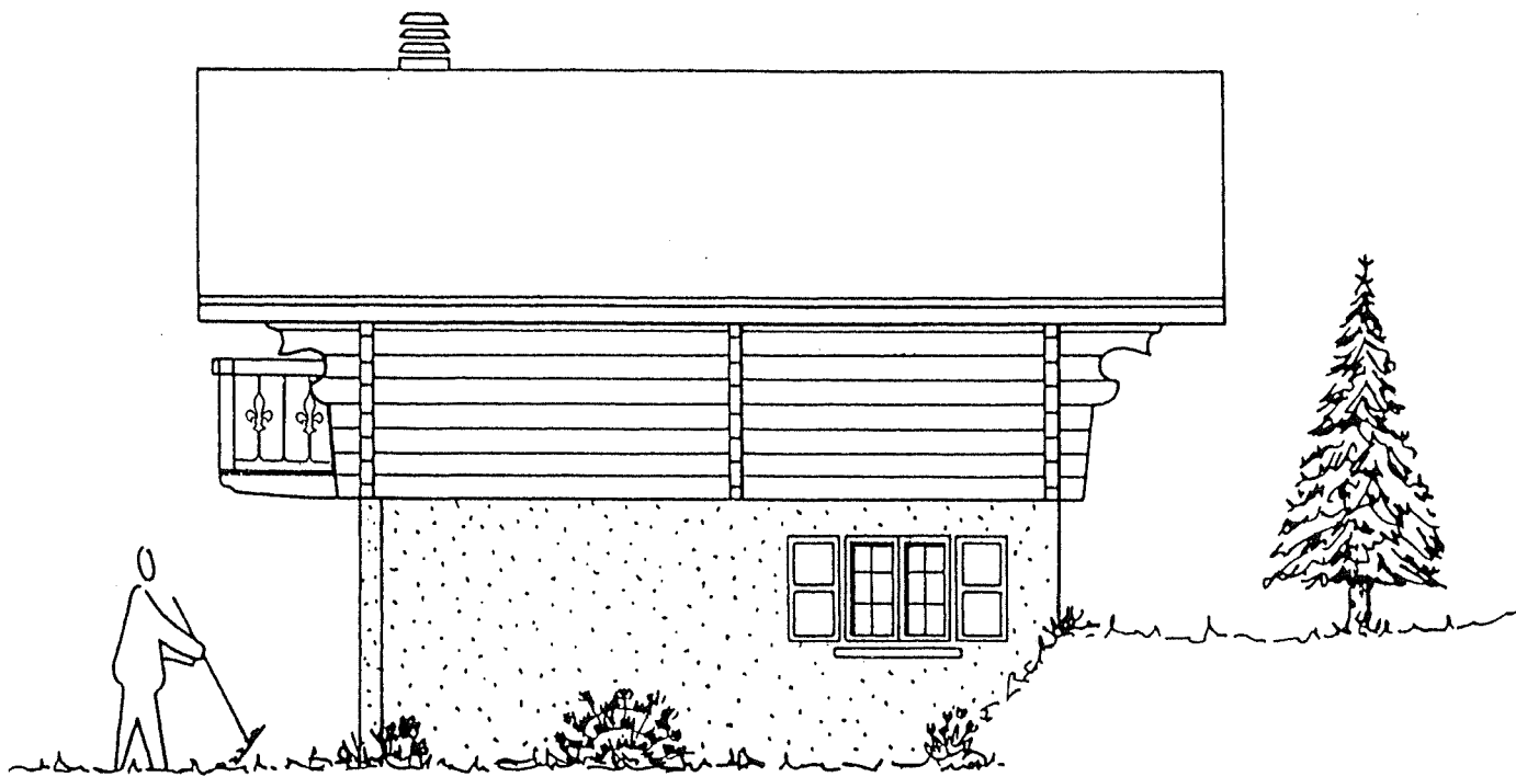
FAÇADE EST
