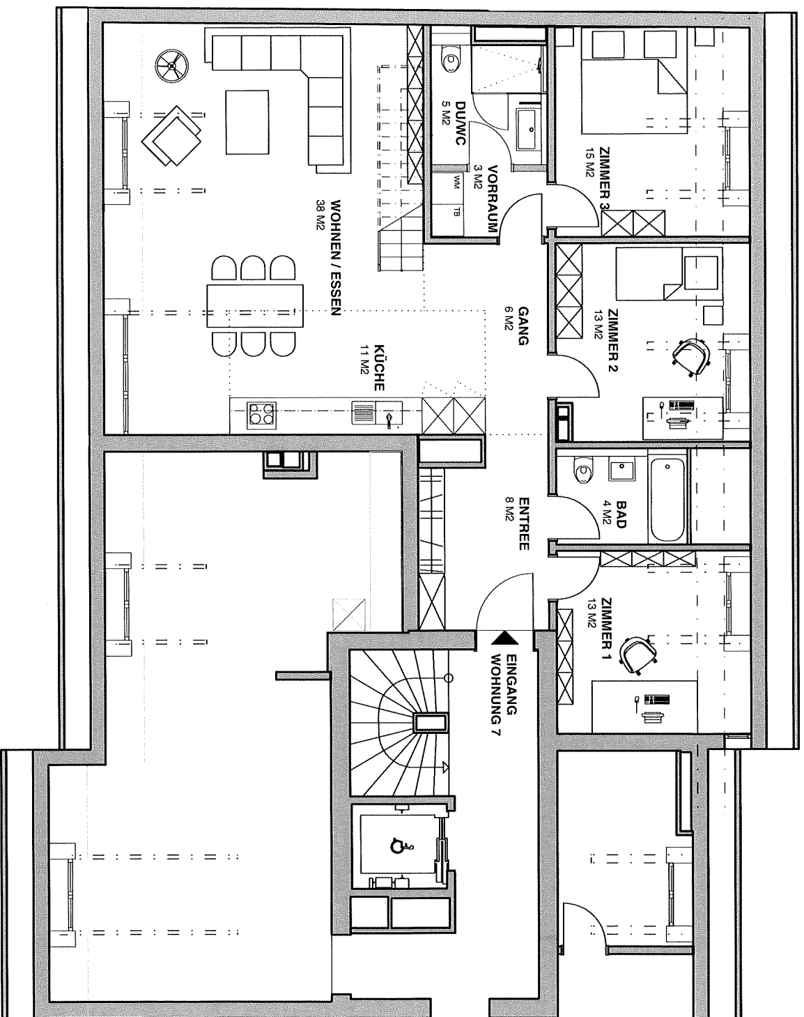
3.OG, Wohnung Nr. 7 159 m²
