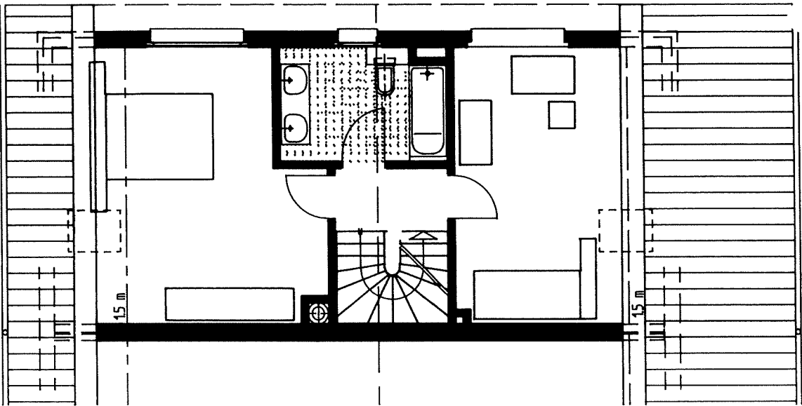
Dachgeschoss
