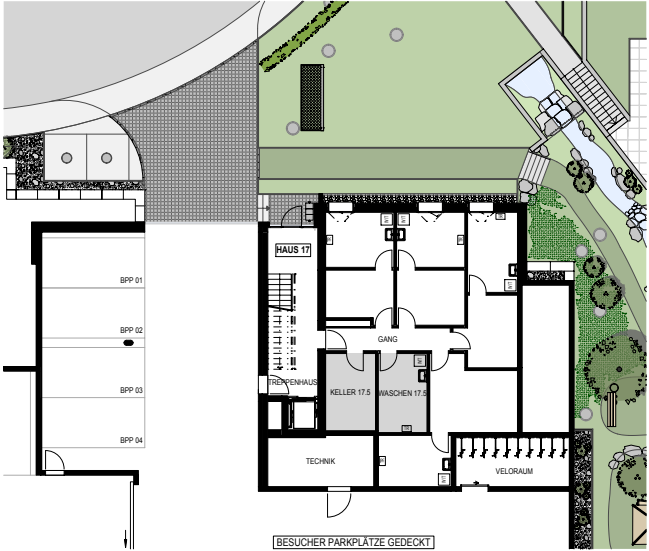
UNTERGESCHOSS 1:400
