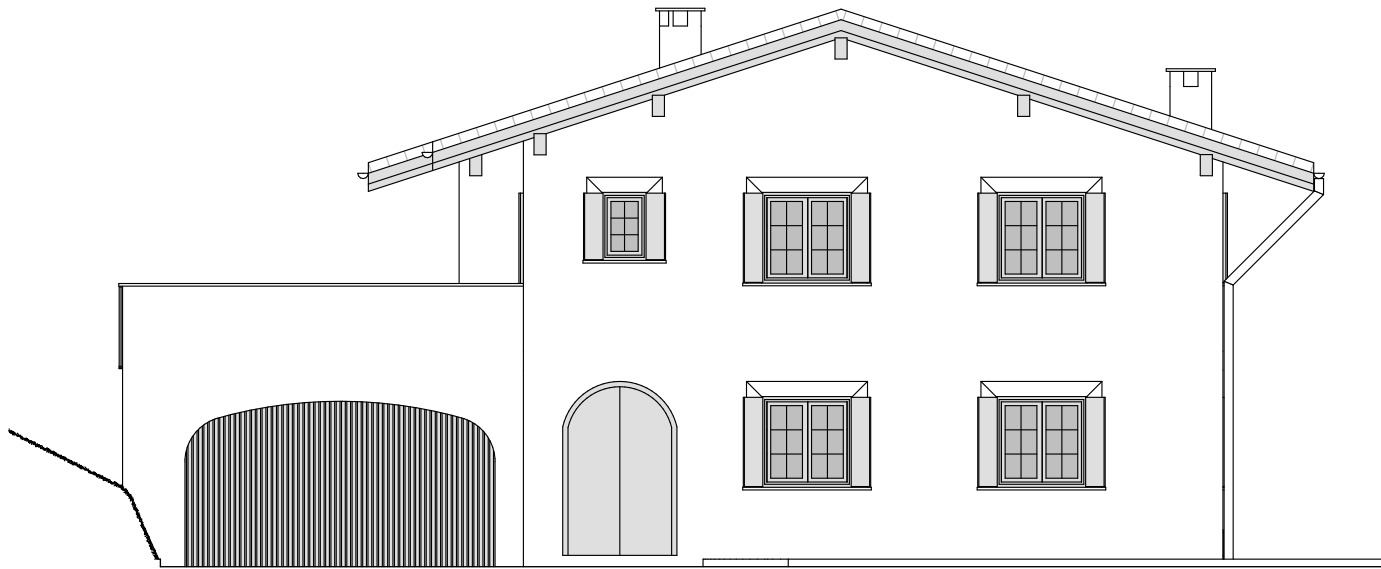
Ansicht Norden / 1:100
