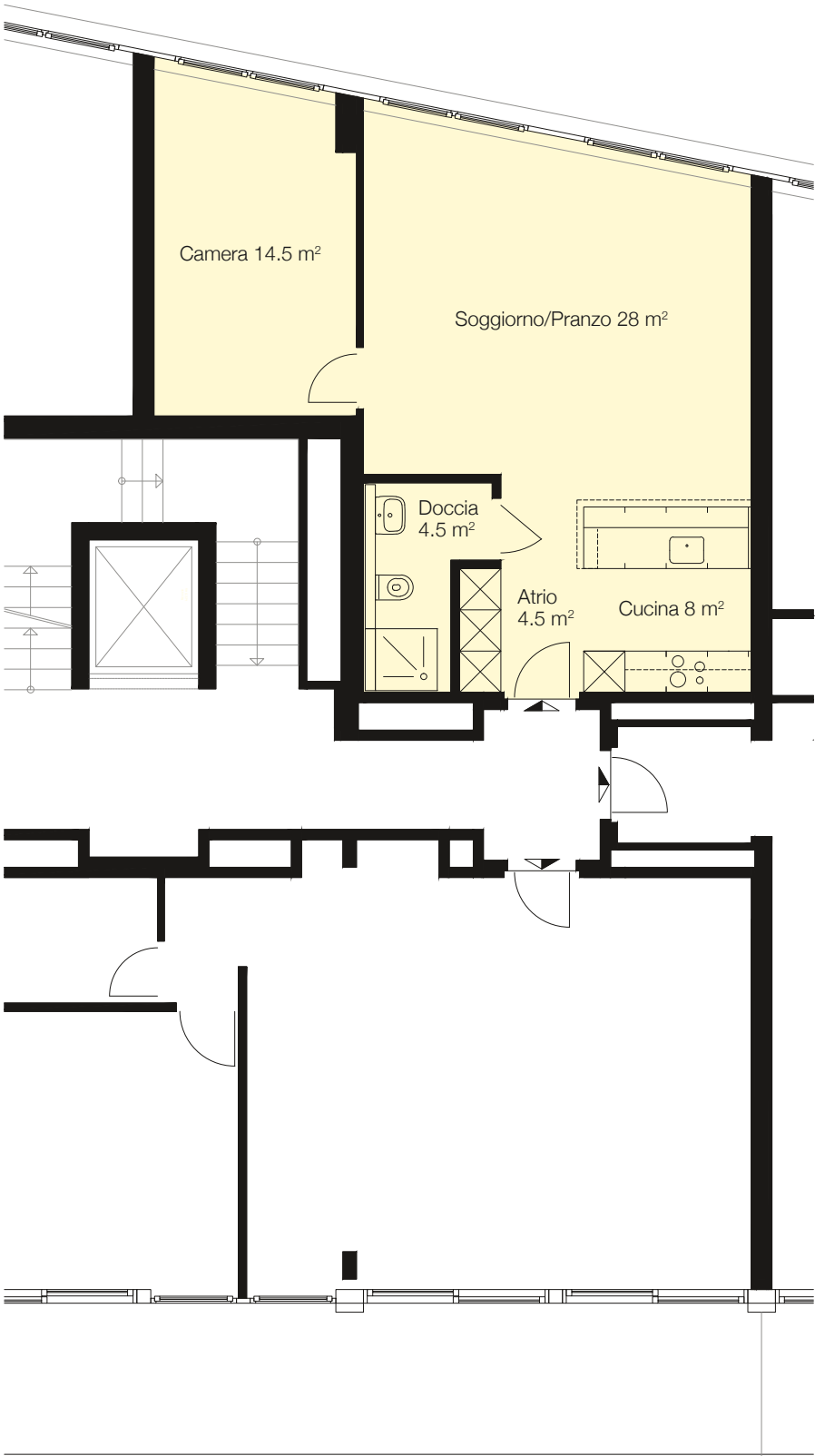
Pianta Scala 1:100
