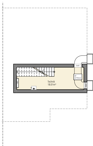
Untergeschoss
