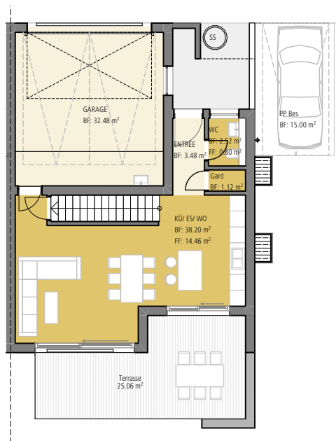
Erdgeschoss
