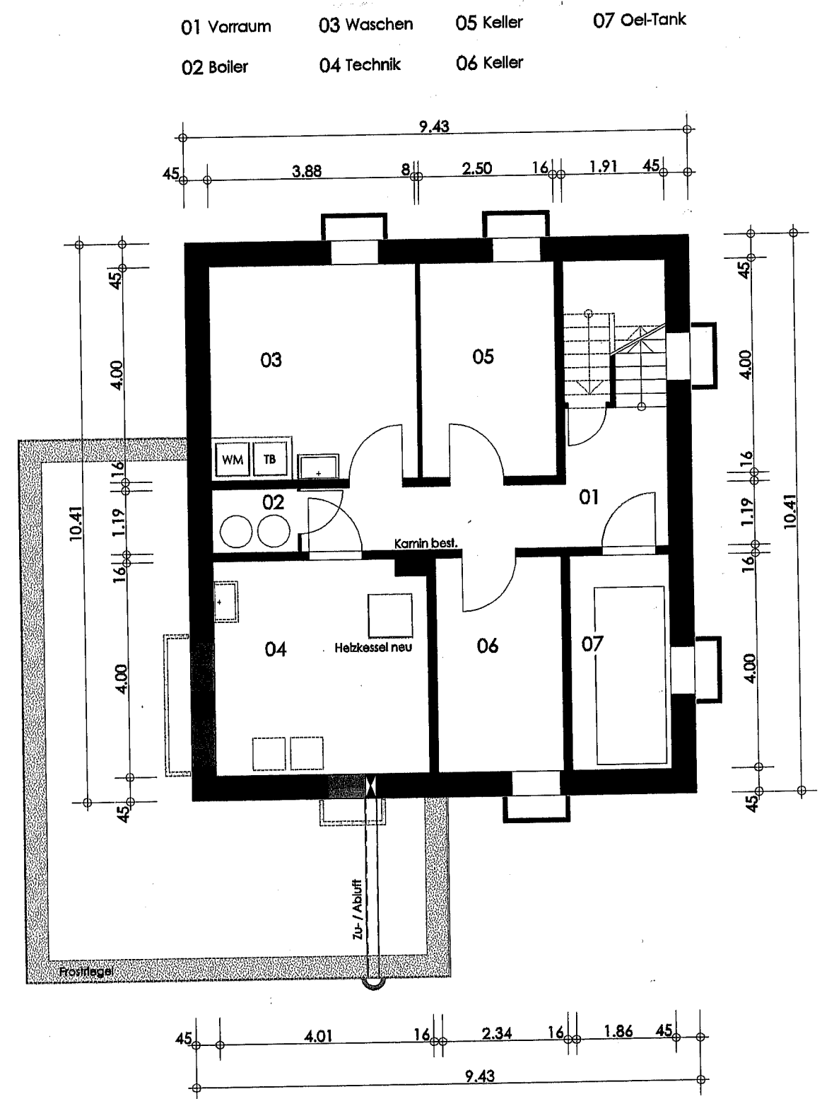
Untergeschoss
