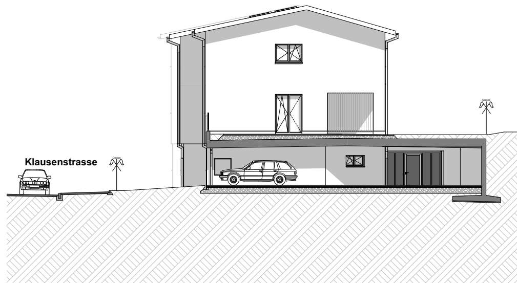
Ansicht West DEFH 1
