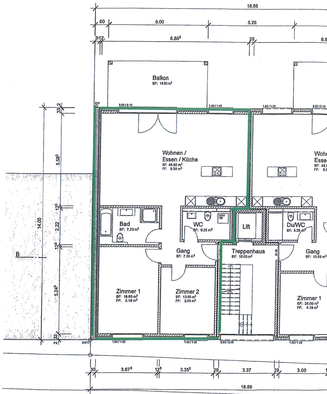
1. - 3. Obergeschoss
