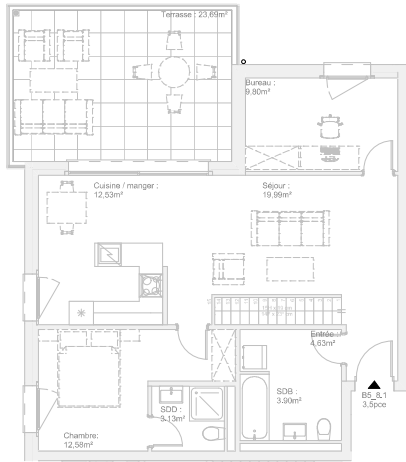
Etage 2: 1:100
