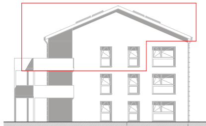
Façade Est : 1:200
