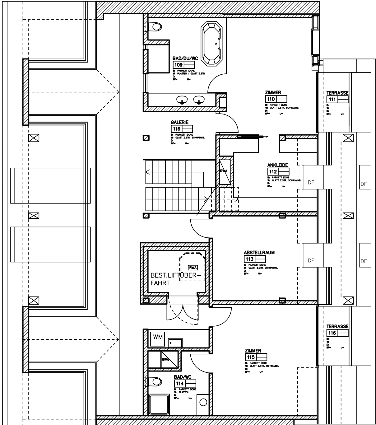
Objekt: Hotel Alpina, Frankenstrasse 6, 6003 Luzern GRUNDRISS DACHGESCHOSS 1:50
