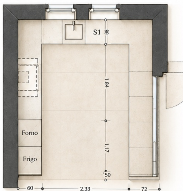
CUCINA - PIANTA
