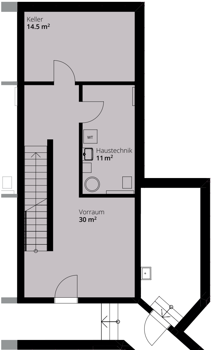
Untergeschoss
