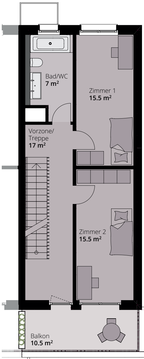
1. Obergeschoss
