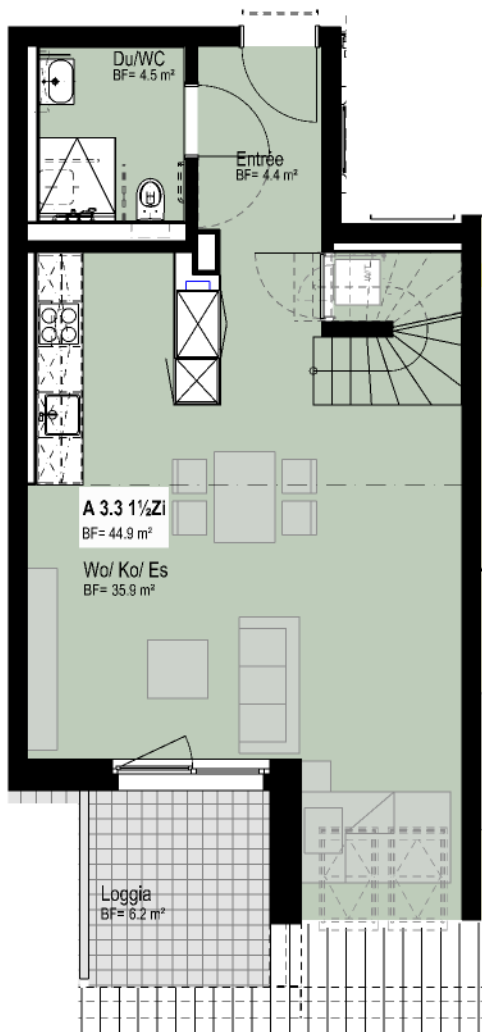
1.Dachgeschoss 44.9 m²
