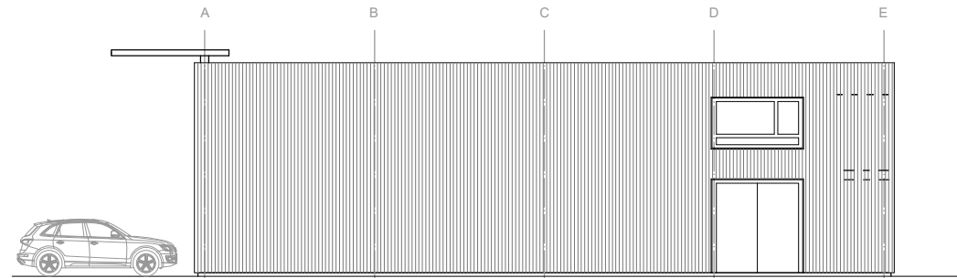
WESTFASSADE
