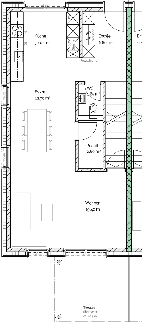
Erdgeschoss
