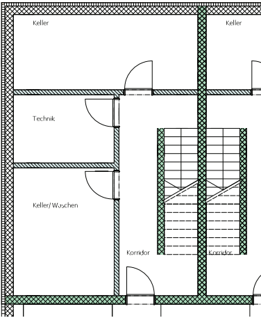
Untergeschoss
