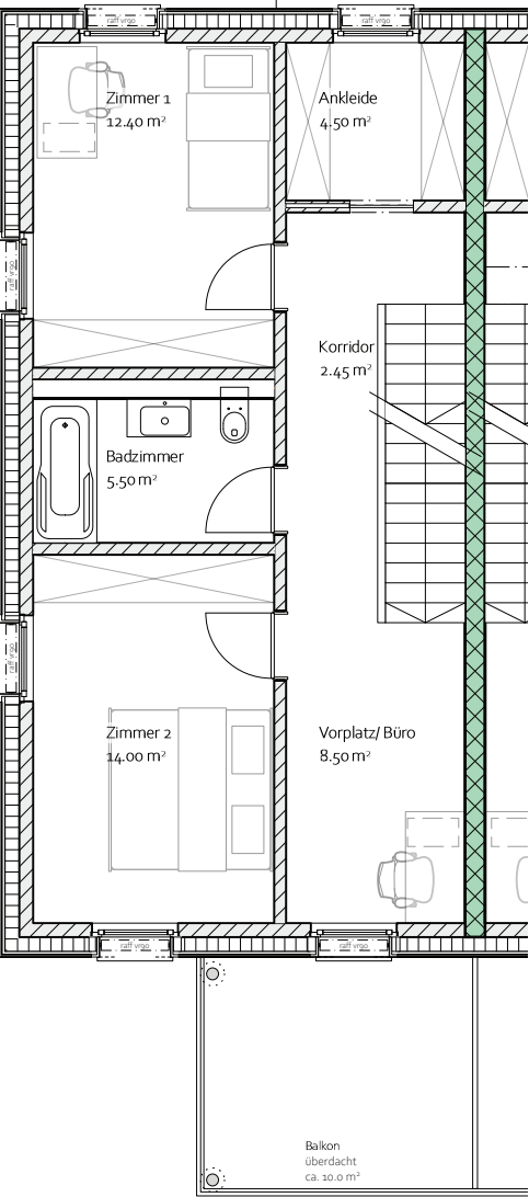
Obergeschoss
