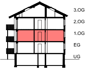
Schnitt
