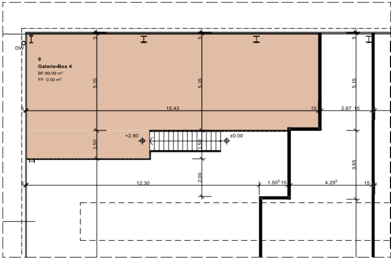
Grundriss Galerie-Box 4 1:100
