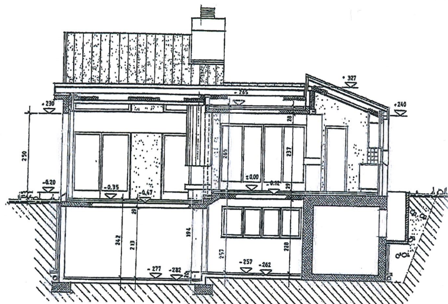
COUPE B-B
