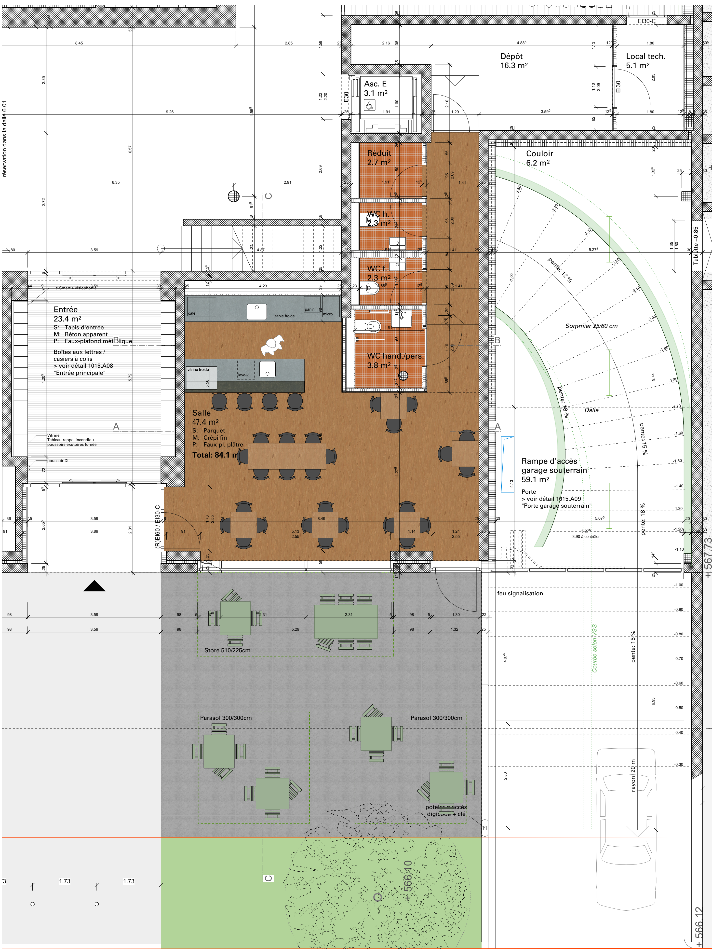
Plan 1:50
