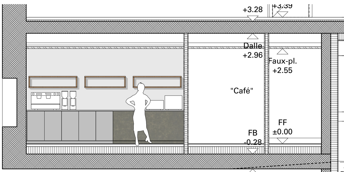
Coupe B-B 1:50
