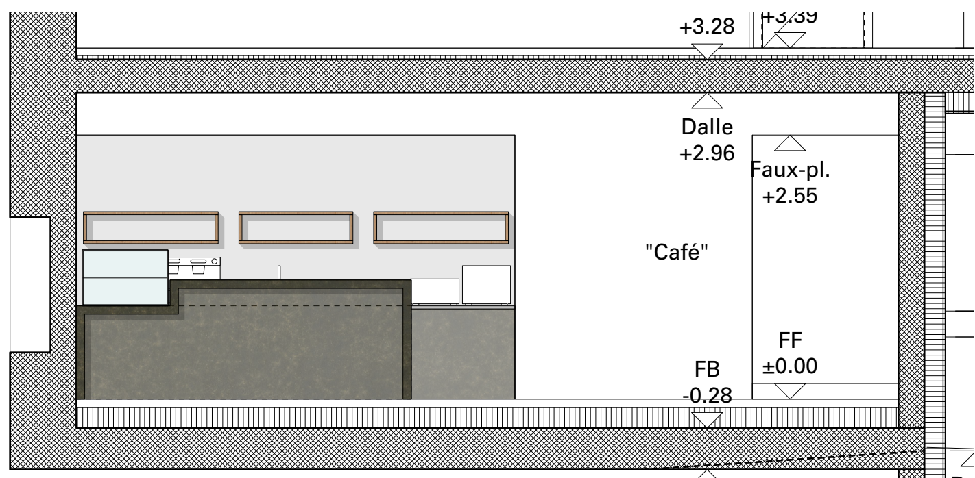
Coupe A-A 1:50
