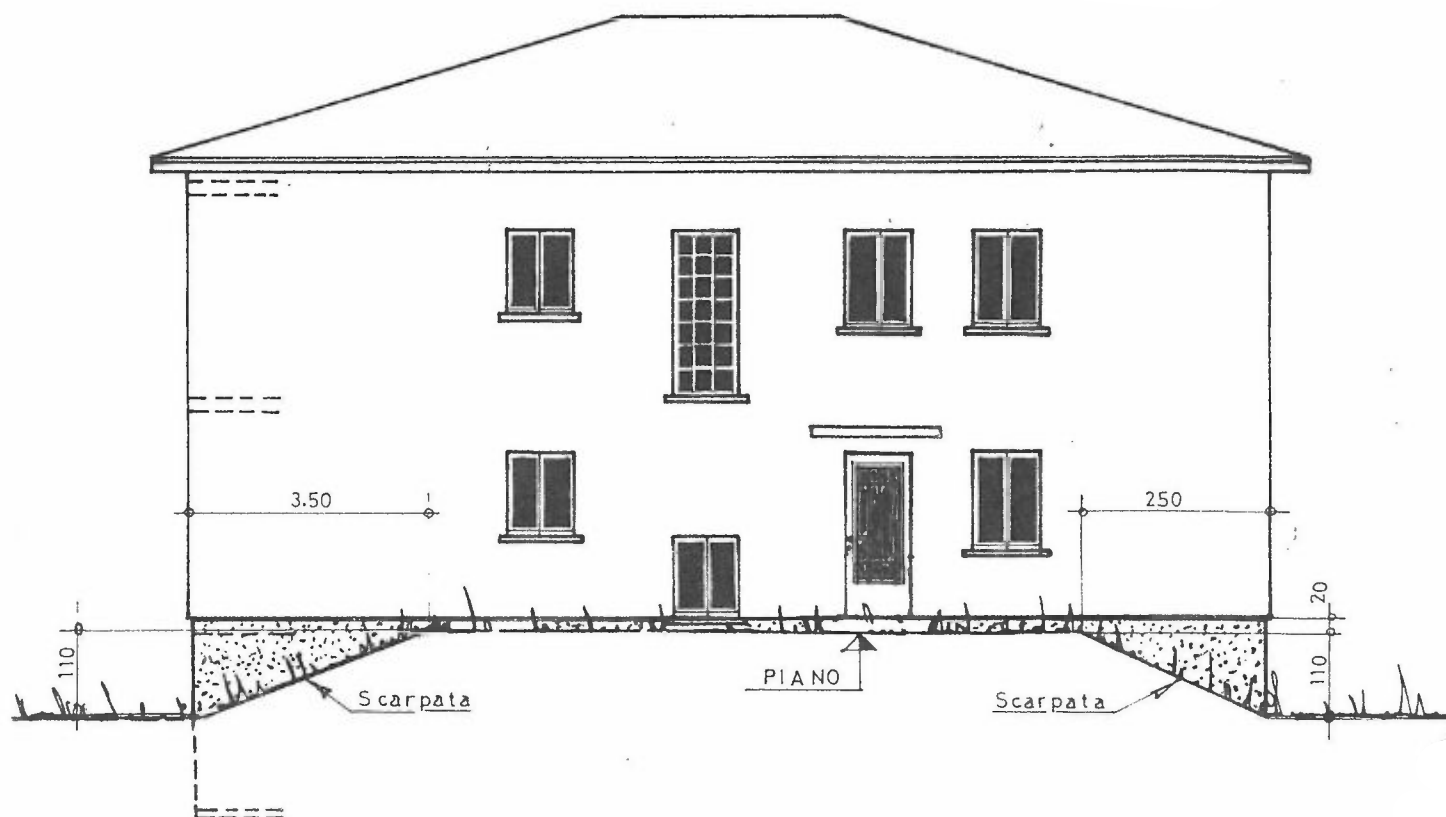
FACCIATA NORD
