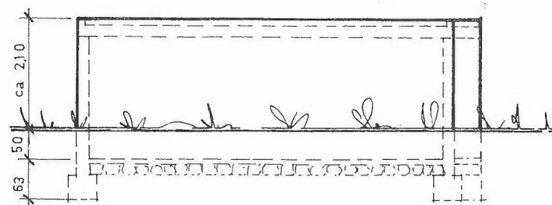
PROSPETTO SUD
