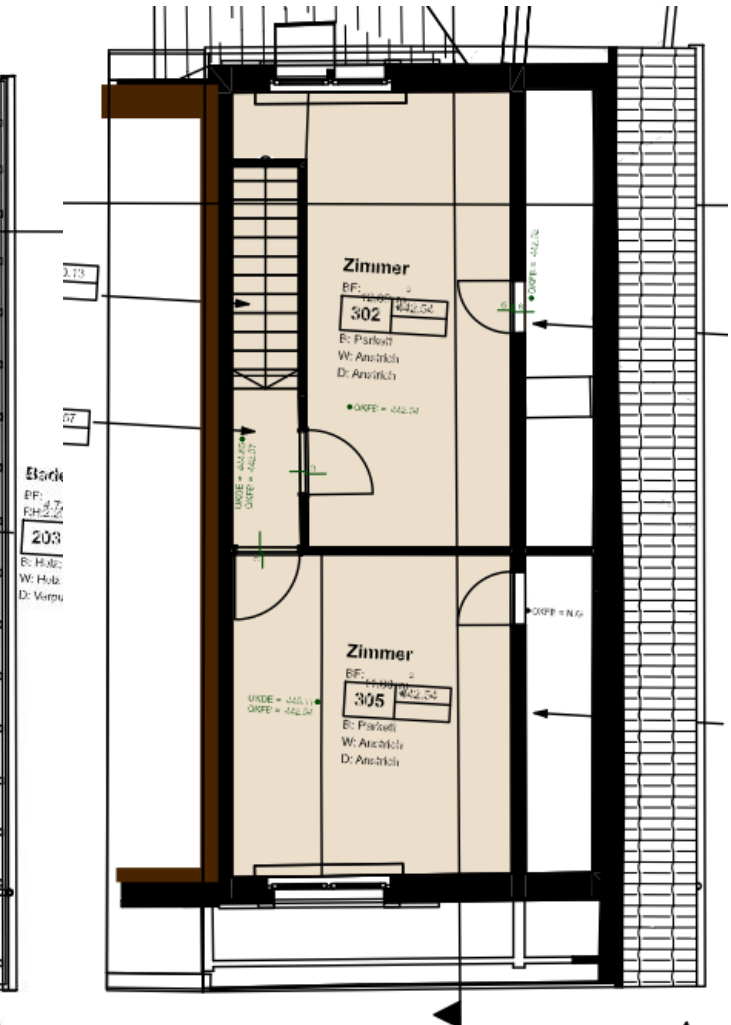
3. Obergeschoss
