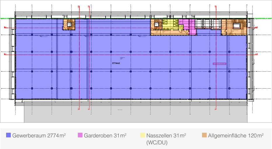
1. Obergeschoss
