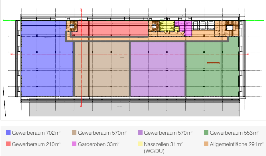
Variante 2. Obergeschoss
