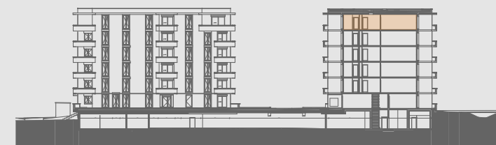
Coupe générale
