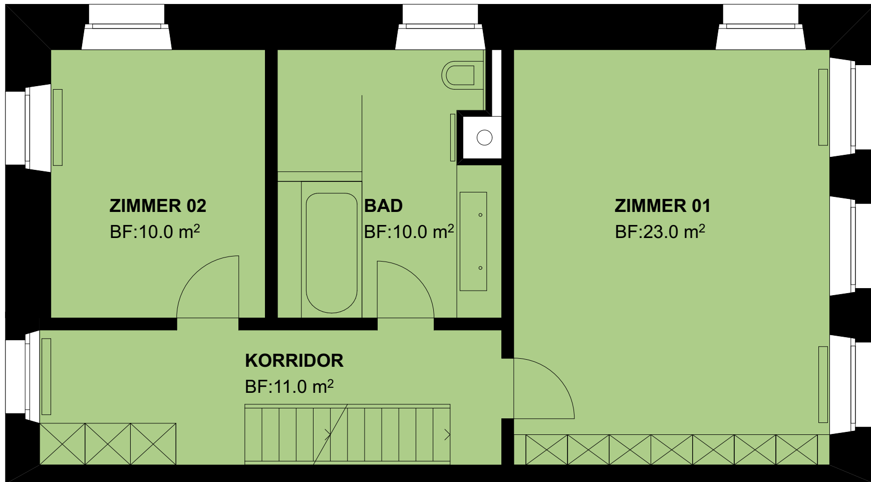
Obergeschoss
