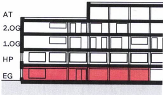
Schnitt
