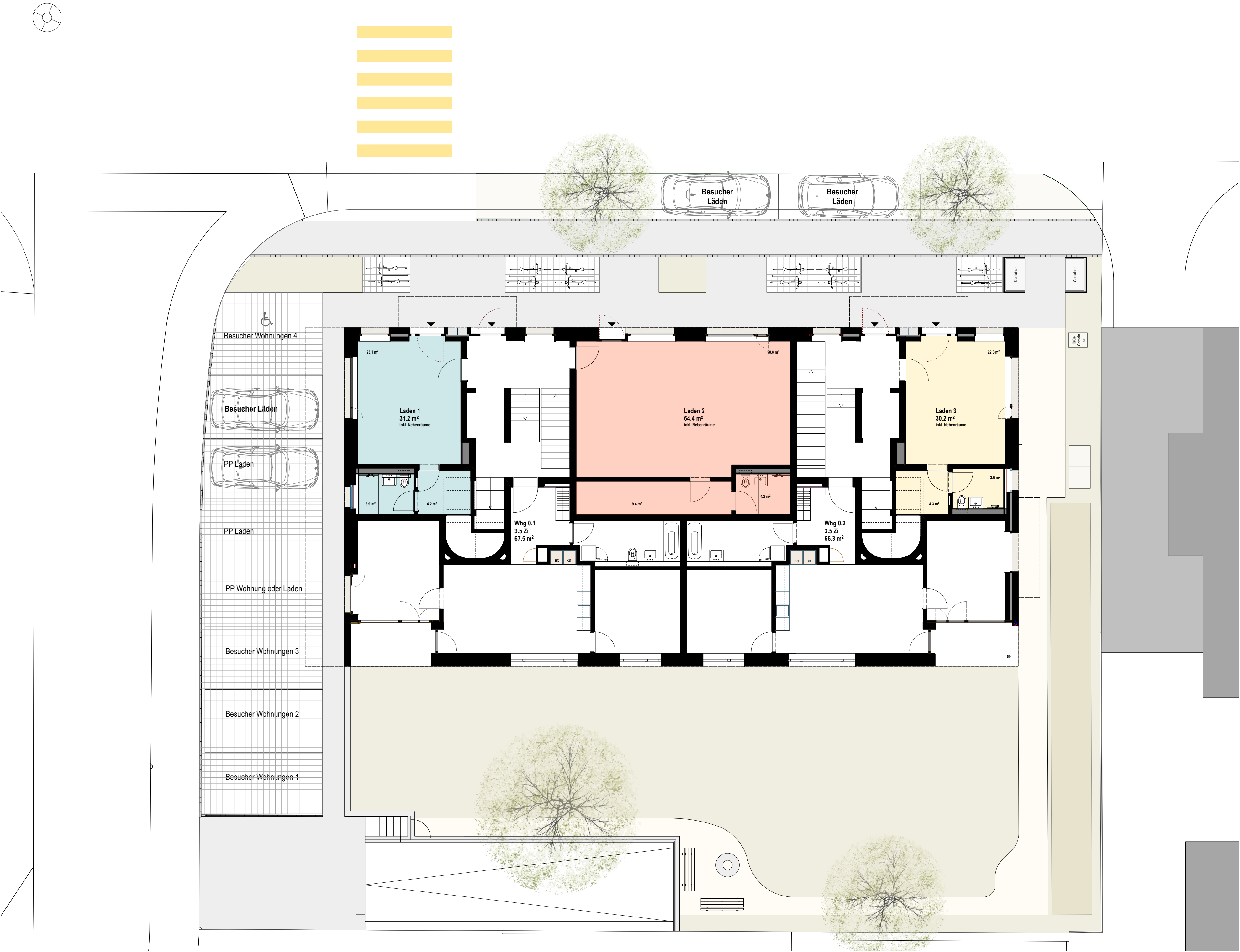
Grundriss Erdgeschoss mit Umgebung
