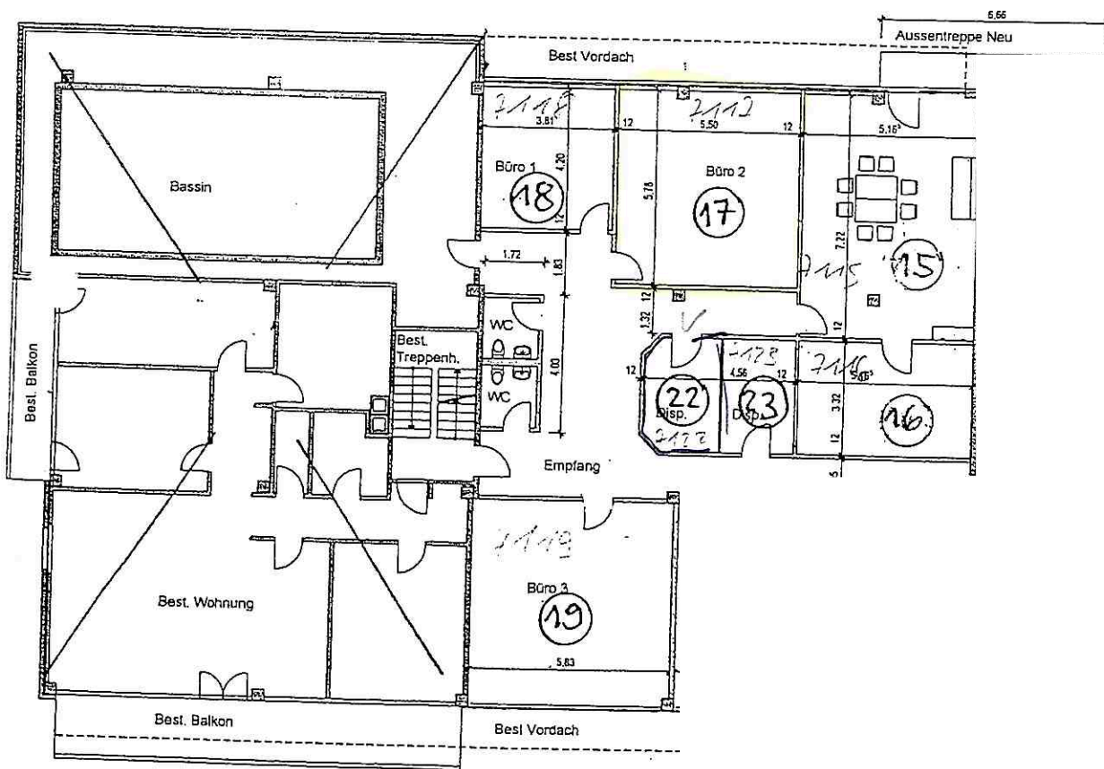
OBERGESCHOSS
