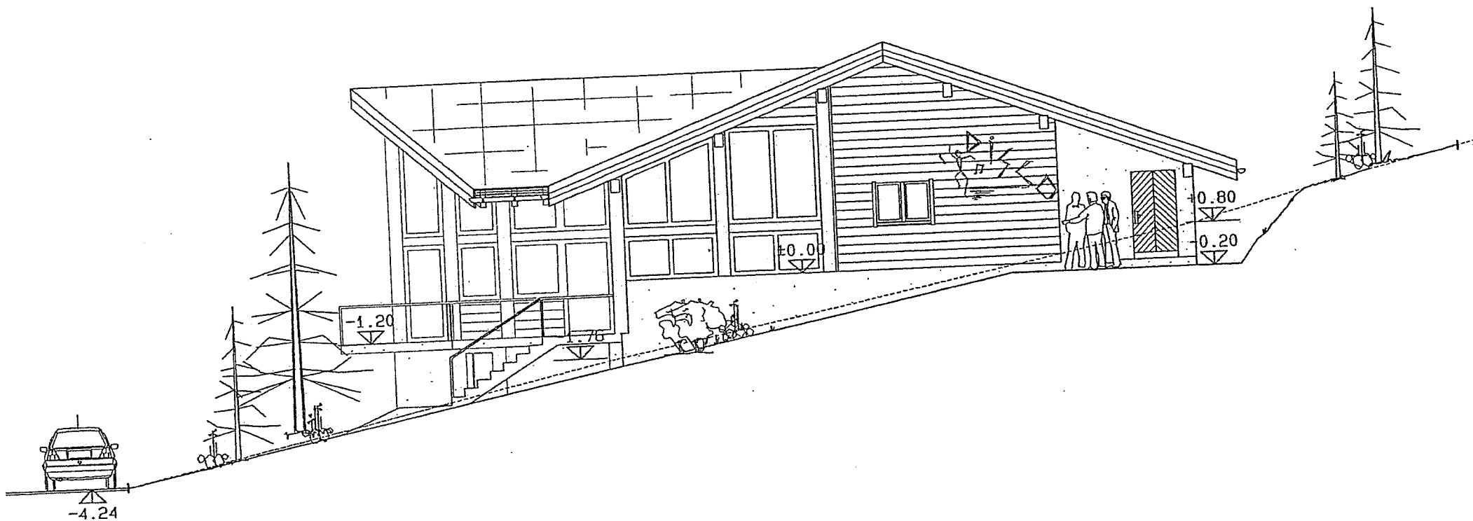
NORD- WESTANSICHT
