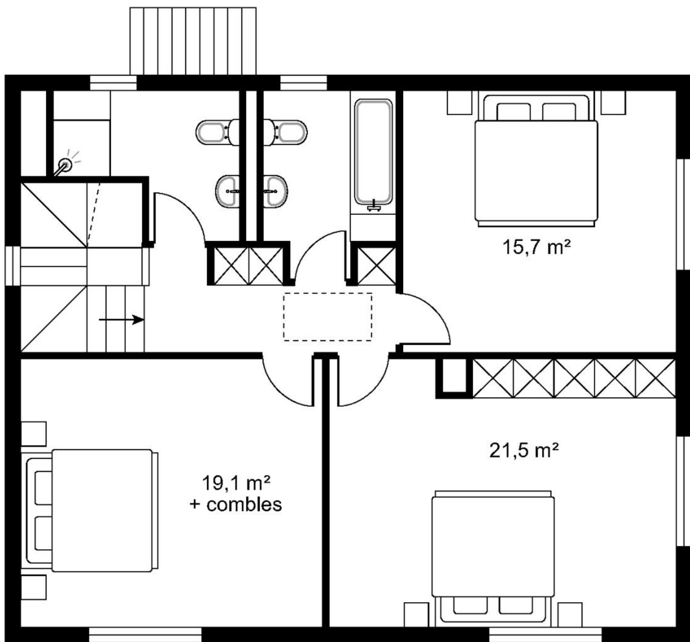
1ER ETAGE
