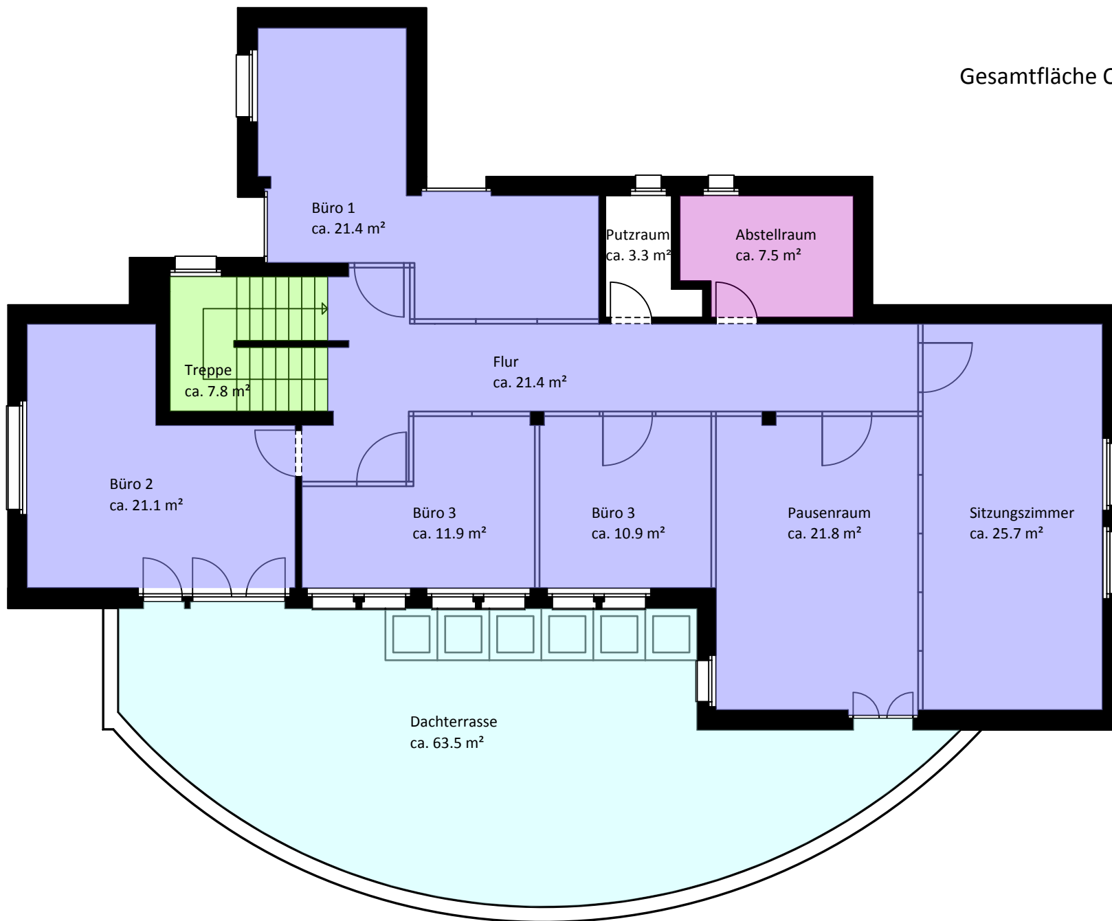
Grundriss Obergeschoss Talackerstrasse 89, Winterthur
