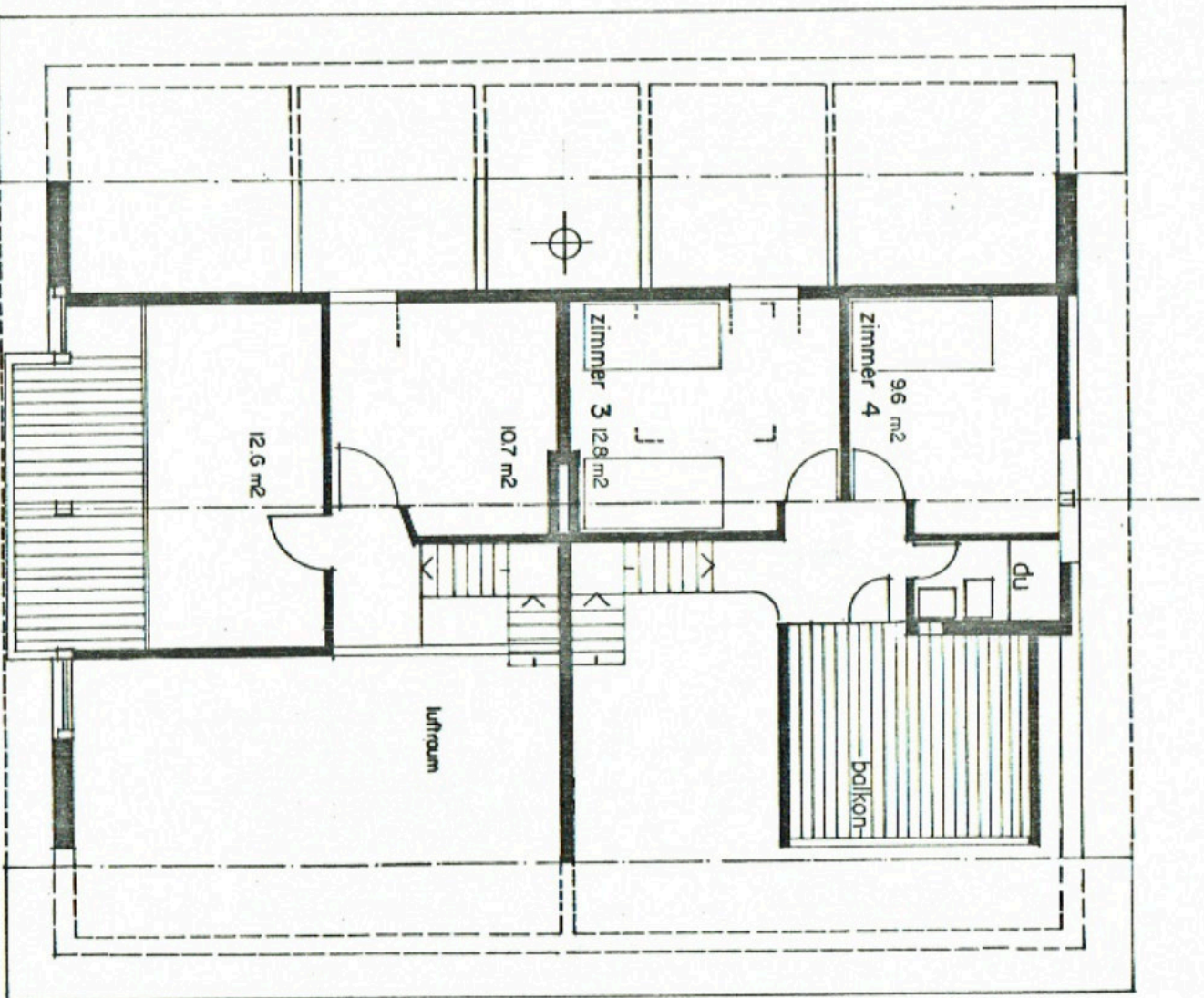
dachgeschoss 1:100
