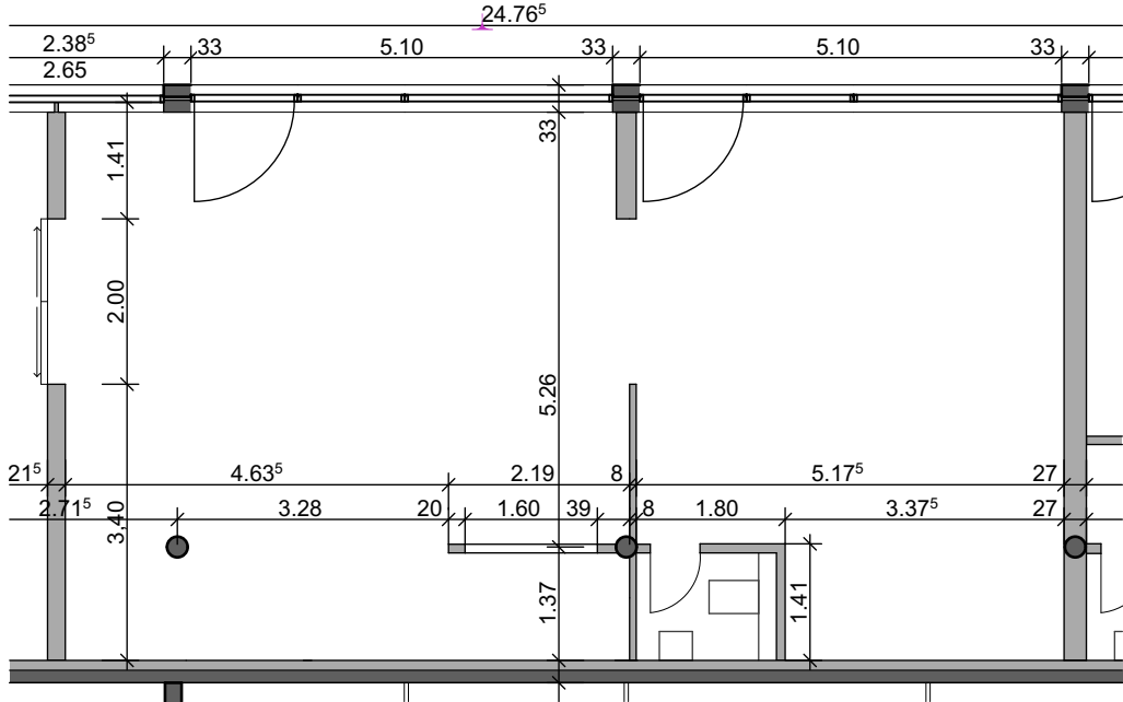
Erdgeschoss
