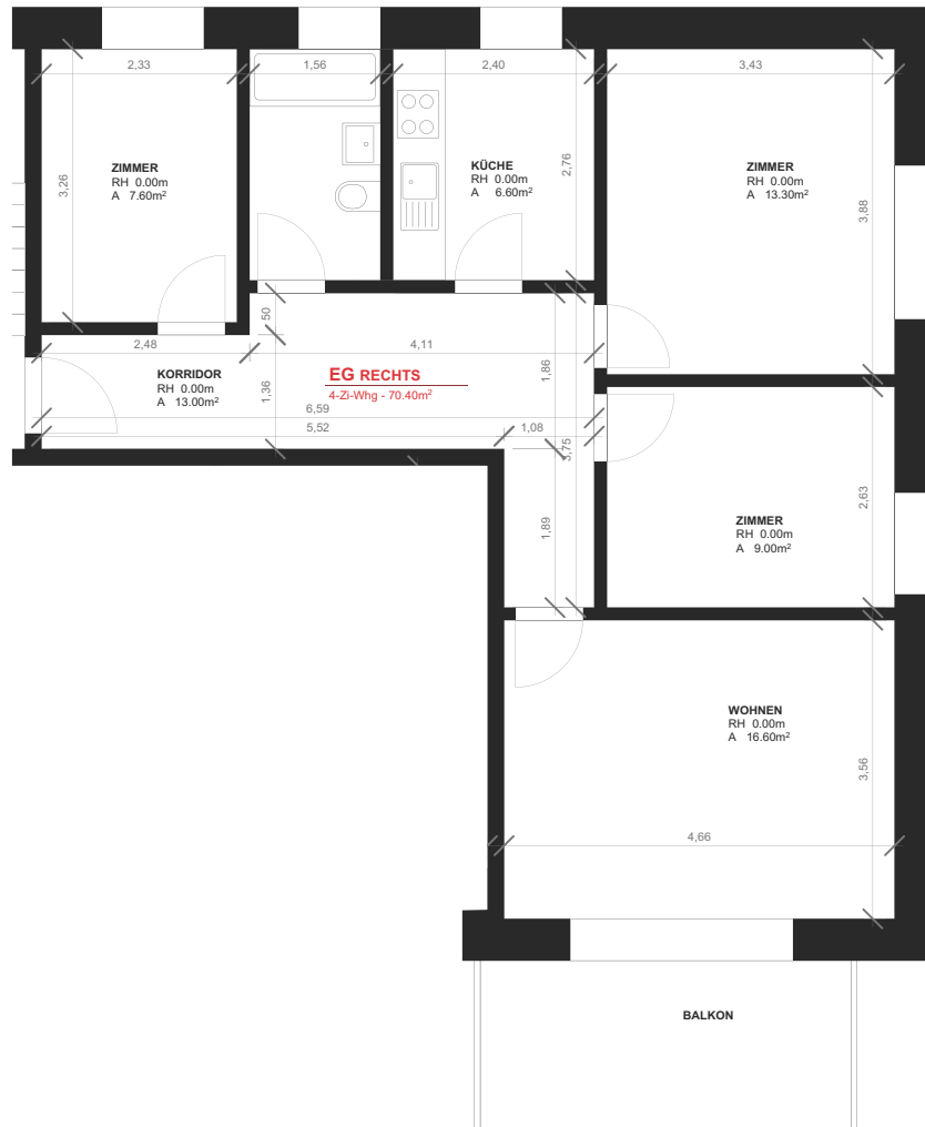
WOHNUNGSGRUNDRISS, 1:100
