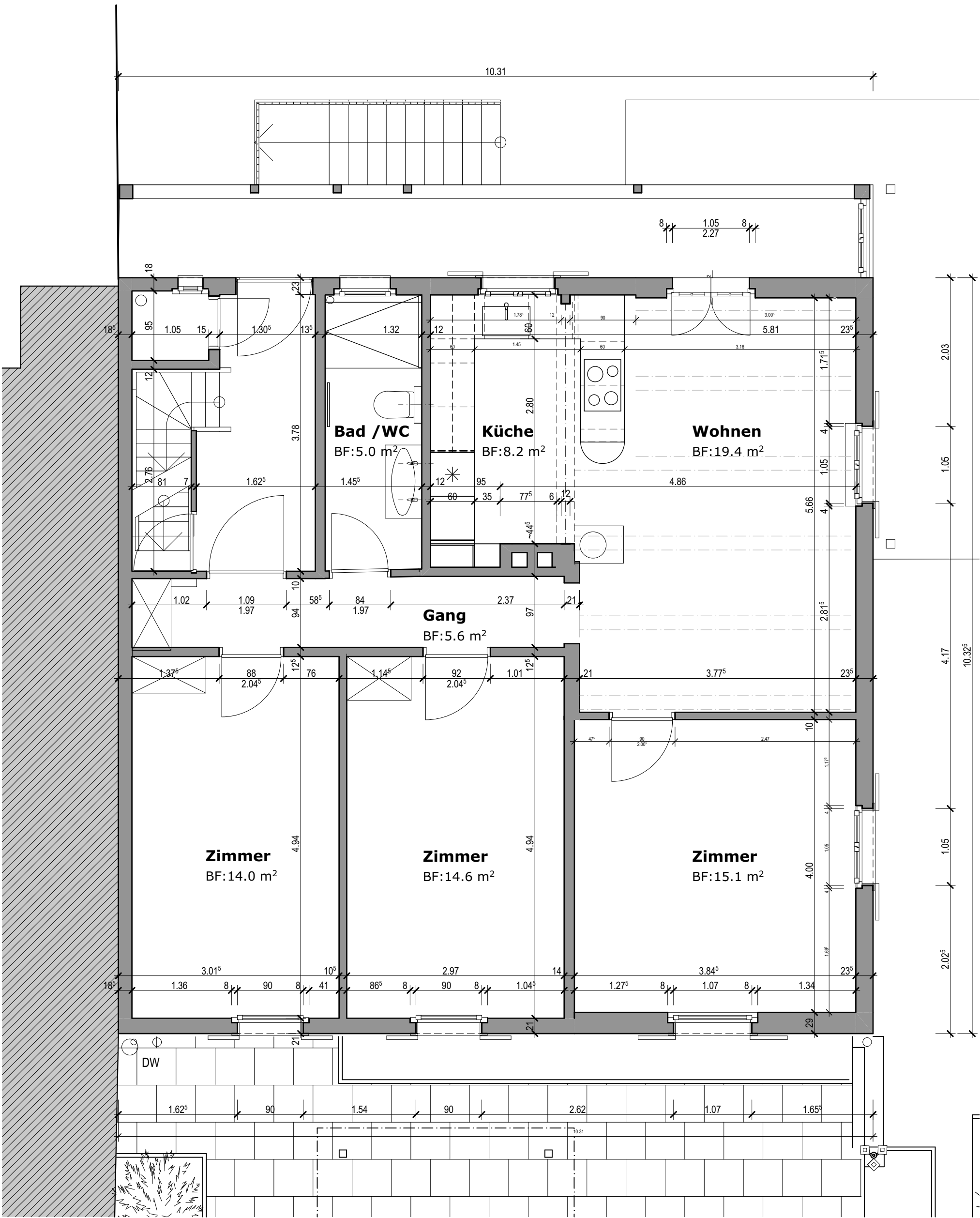
Pl. Nr.: 140-402 ERDGESCHOSS
