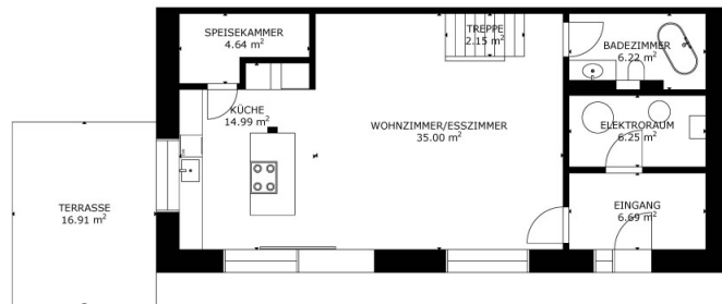
ERDGESCHOSS
