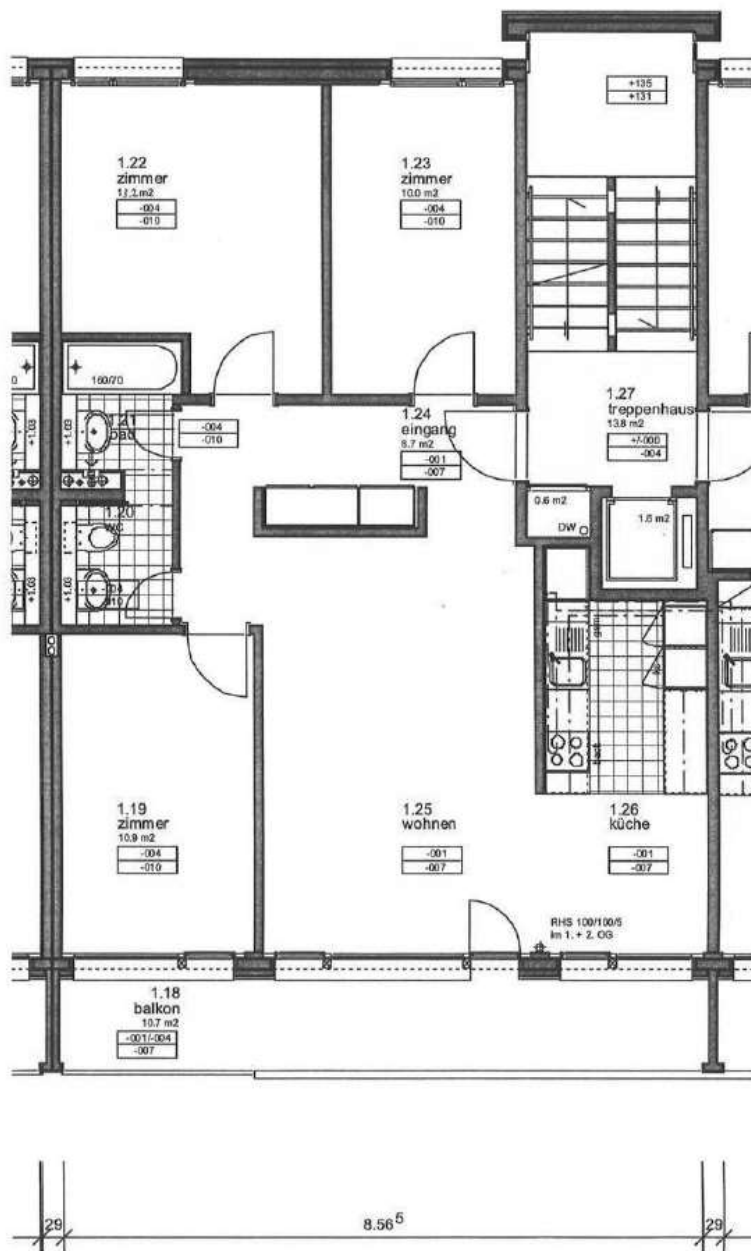
Grundriss Typ B 1.- 4. OG
