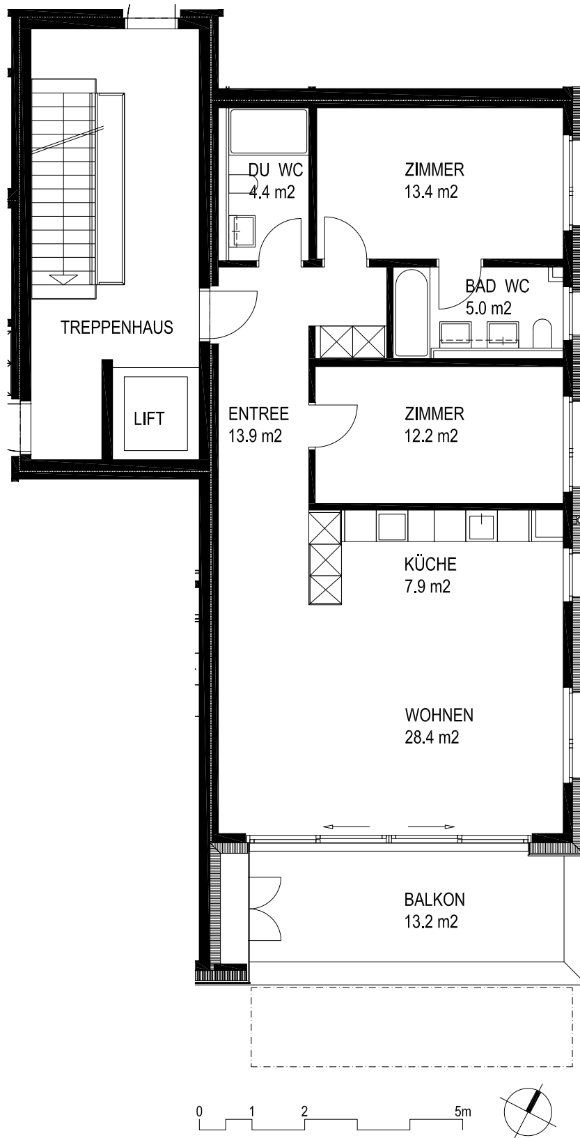
Wohnung B1/B3/B5-13/23/33/43
