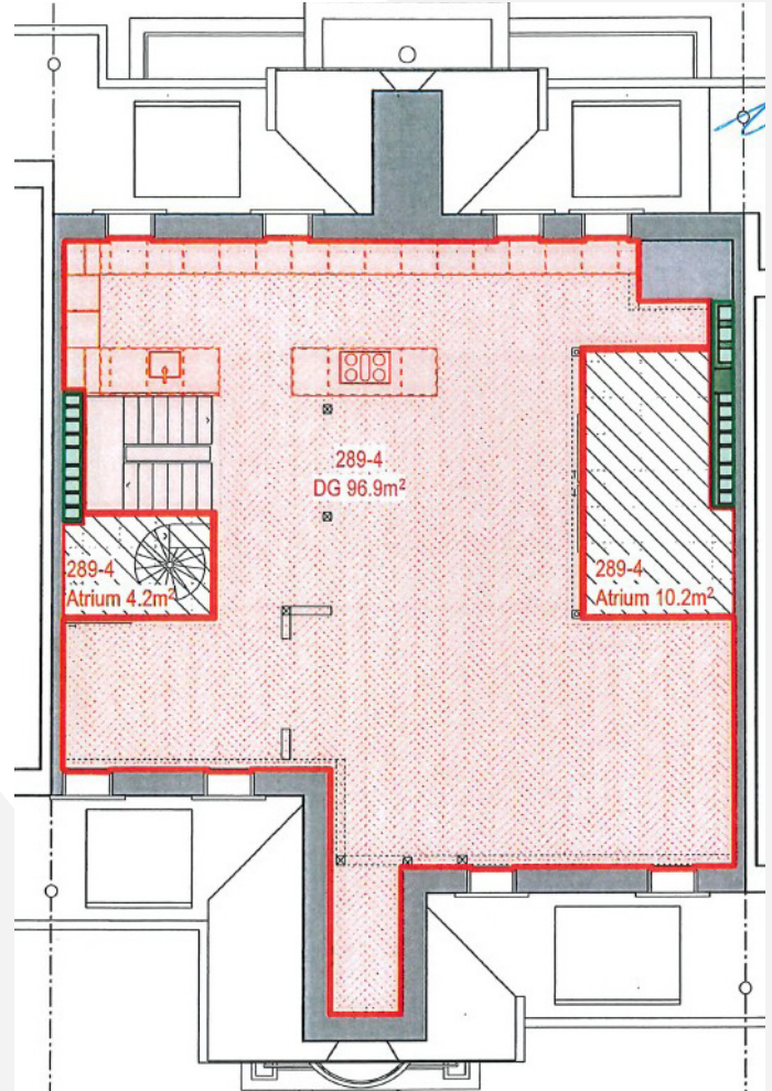
2. Geschoss der Maisonettewohnung
