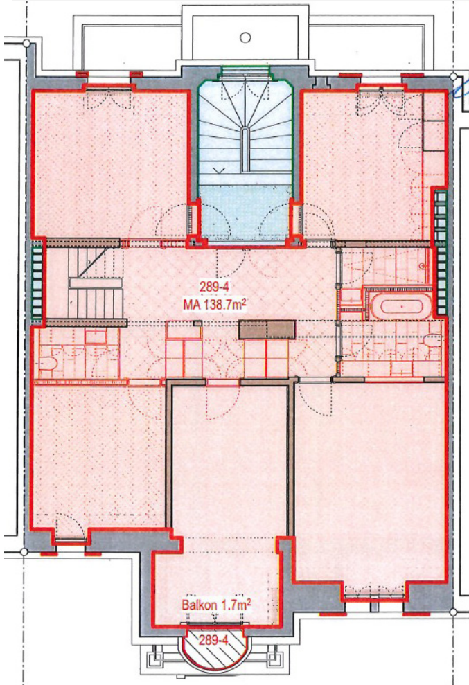
1. Geschoss der Maisonettewohnung
