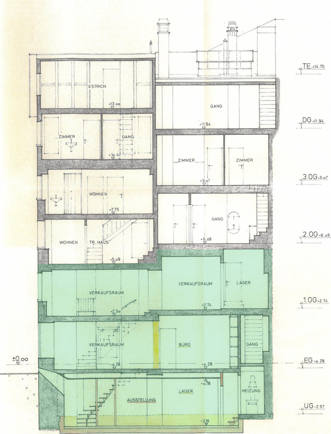
SCHNITT A-A
