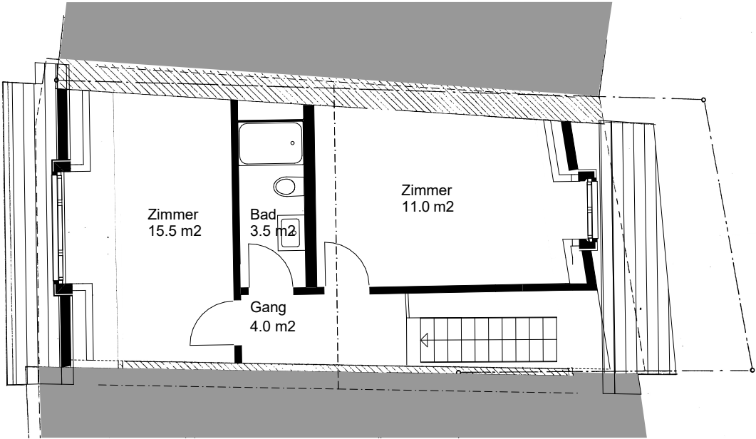
GRUNDRISS DACHGESCHOSS
