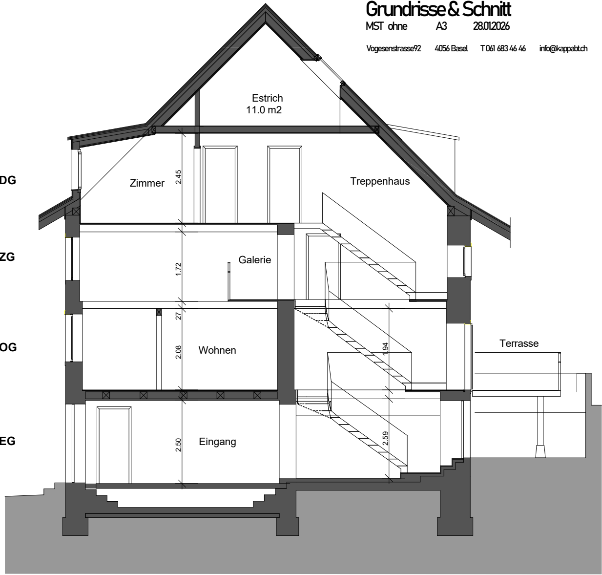
QUERSCHNITT
