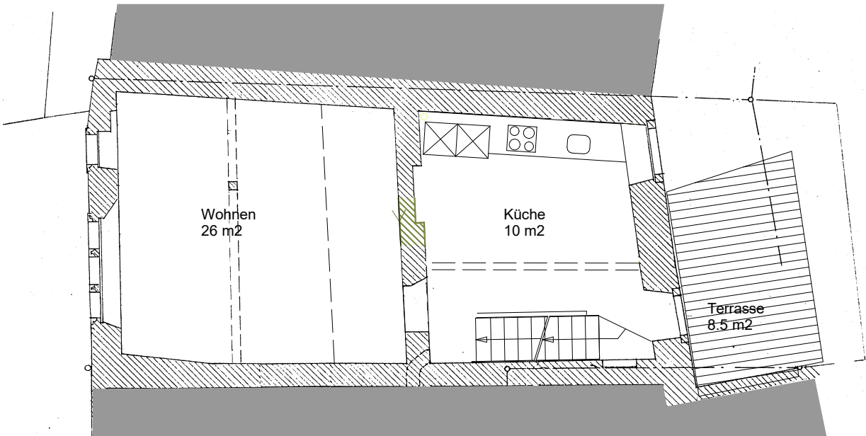
GRUNDRISS OBERGESCHOSS
