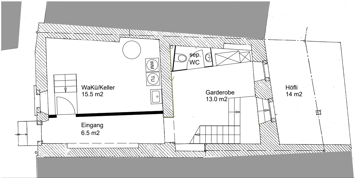
GRUNDRISS ERDGESCHOSS
